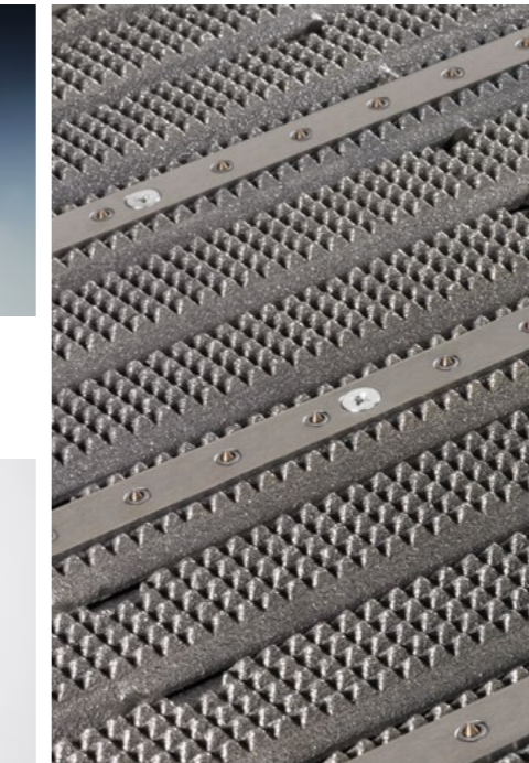
Spikes: seitliche Führung für exakte Parallelität auch bei verzogenen Hölzern
