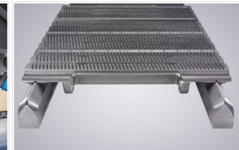
Prismengeführte Vorschubkette: beste Schnittergebnisse
